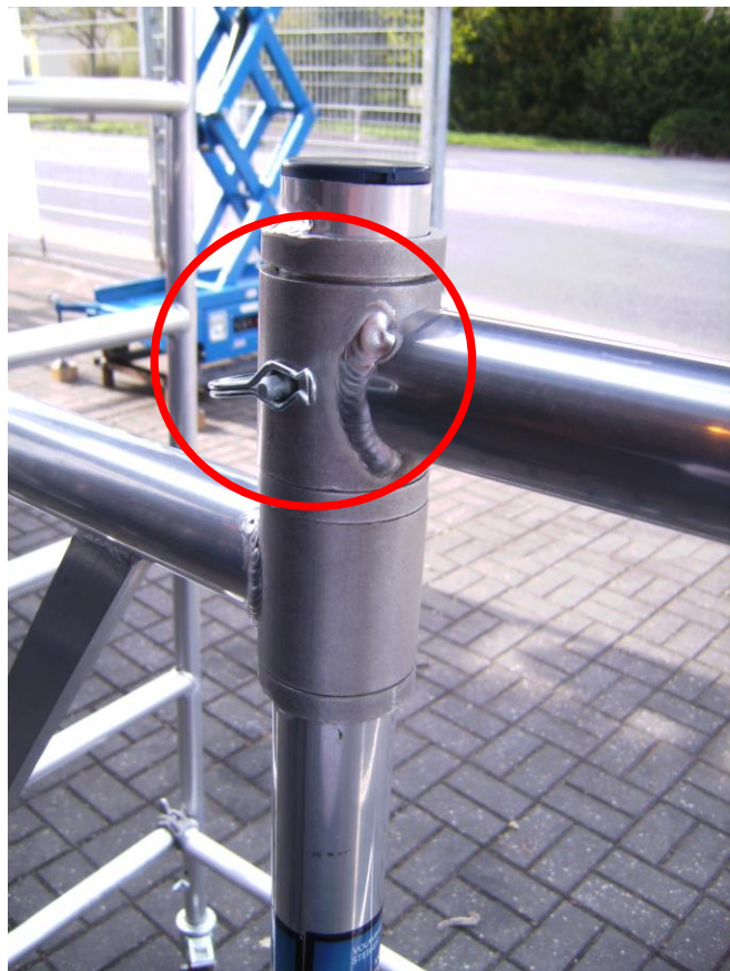
Sicherung Klappmechanismus
